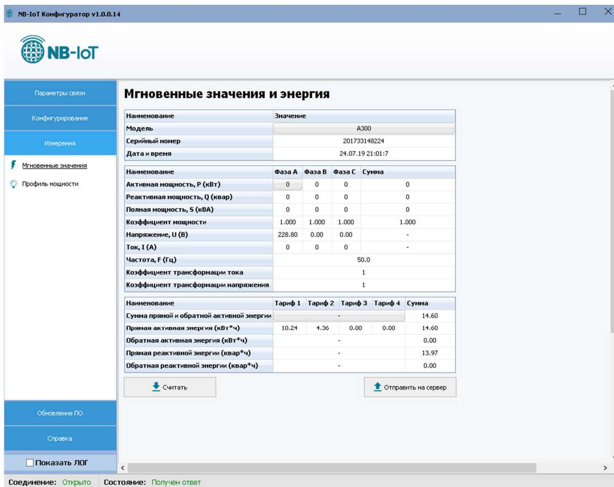
Рисунок 8 – Вкладка «Мгновенные значения и энергия» configurатора
